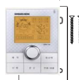
Пульт управления в комплекте: кронштейн крепления к стене - 1 шт. шуруп M3 x 45 мм - 2 шт
