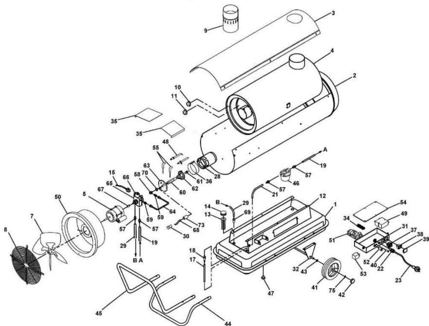
Рис. 1. Разборная схема тепловой пушки
