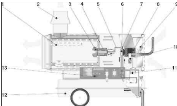
Рис. 2. Принципиальное устройство тепловой пушки 1-камера сгорания, 2-дымовая противоветровая муфта, 3-горелка, 4-сопло, 5-топливная цепь, 7-электроклапан топлива, 8-мотор, 9-вентилятор, 10-ручка, 11-фильтр топлива, 12-топливный бак, 13- блок управления.
