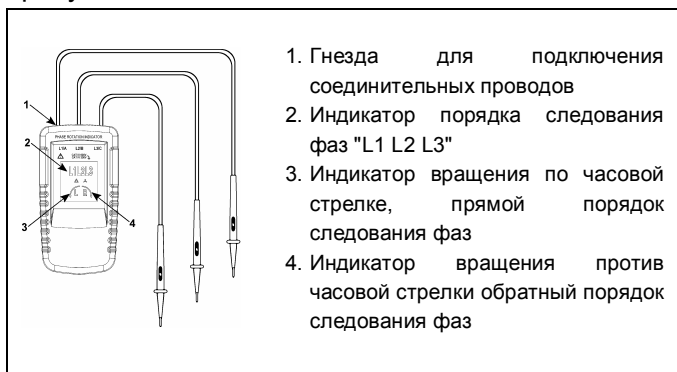
Рисунок 1. Фазоуказатель
