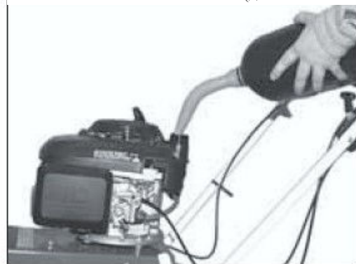
1. Топливный и масляный бак (двигатель Honda)
