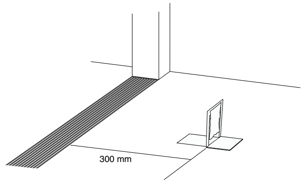
Asetustyökalun sijoitus
