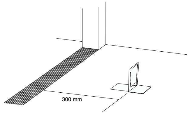
Placering av injusteringsverktyg
