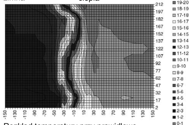
Rozkład temperatury przy prawidłowo wyregulowanej kurtynie
