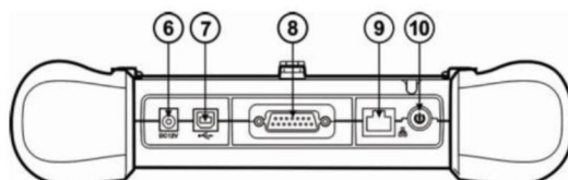
Рисунок 1-3. Сканер MaxiDAS® (вид сверху)
