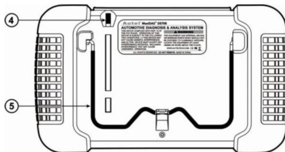
Рисунок 1-2. Сканер MaxiDAS® (вид сзади)
