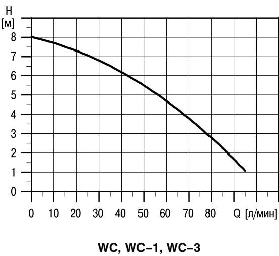
Рабочая характеристика
