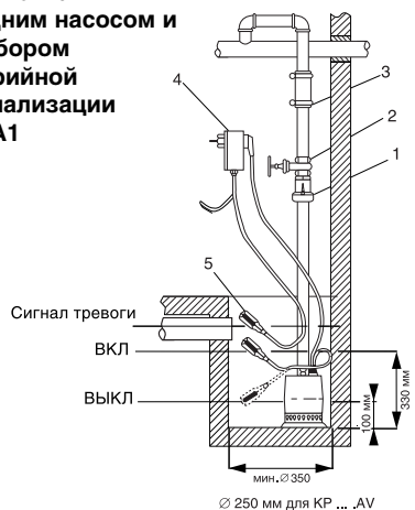
Габариты места установки насоса Unilift KP...AV1
