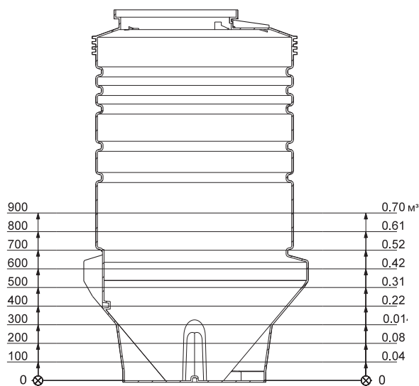
Рис. 13 Полезный объем относительно уровня, PUST 1000 (один насос)
