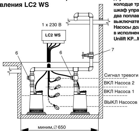
Стационарная установка с двумя насосами и шкафом управления LC2 WS
