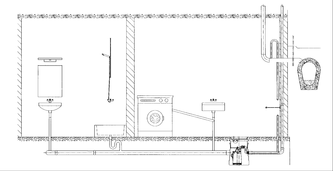
Пример монтажа
