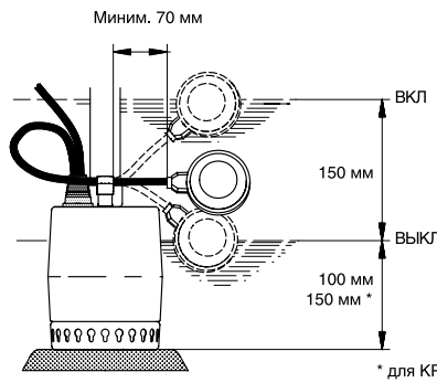
Минимальный уровень включения / выключения
