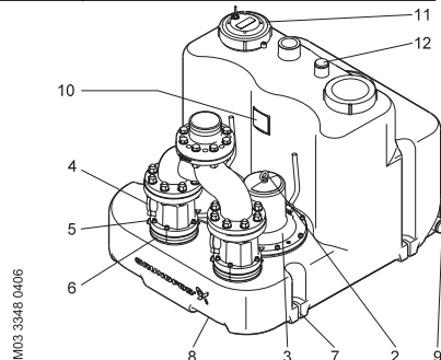
Multilift MLD
