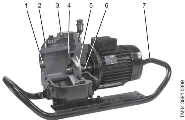
Рис. 3 POMONA PO23 с электродвигателем на раме для переноски
