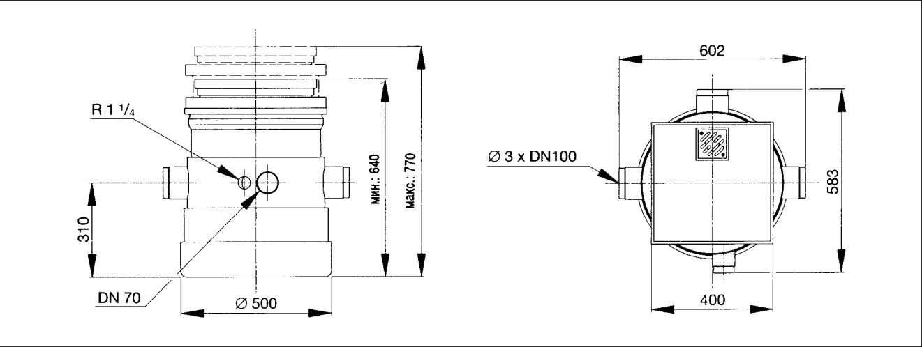
Габаритный чертеж установки Liftaway B
