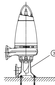
Вертикальная сухая установка
