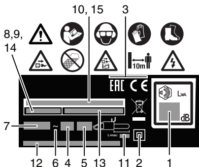
Identifikavimo etiketės pavyzdys
