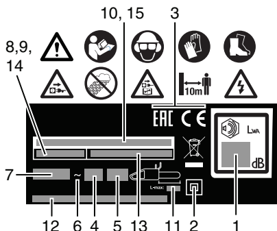
Primjer naljepnice s podacima
