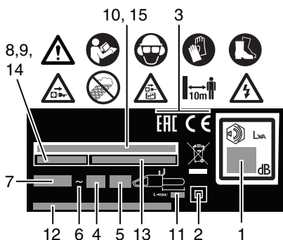
Przykład tabliczki znamionowej wyrobu
