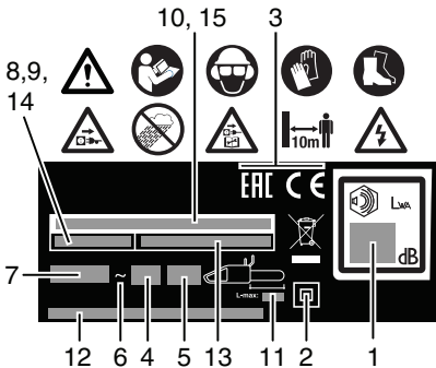
Beispiel für Kennschild
