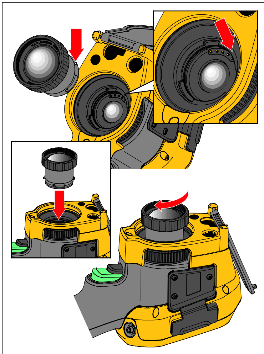
Рис. 2. Установка дополнительного объектива
