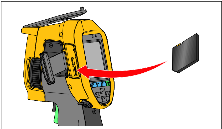
Рис. 3. Вставка и извлечение карты памяти Micro SD
