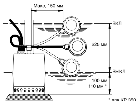
Максимальный уровень включения / выключения
