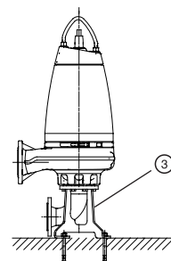
Вертикальная сухая установка
