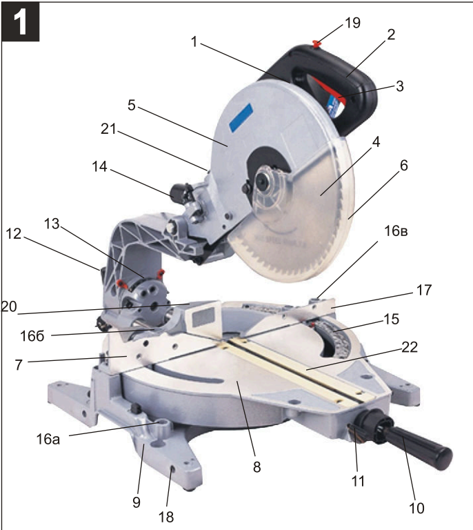
1. Рычаг фиксации подвижного кожуха; 2. Рукоятка; 3. Пусковое устройство; 4. Пильный диск; 5.Основной кожух; 6. Подвижный защитный кожух; 7.Левый упор; 8.Поворотное основание; 9. Стационарное основание; 10. Фиксирующая рукоятка; 11. Стопорная защёлка; 12. Ручка фиксации наклонного положения пилы; 13. Шкала наклона пилы; 14. Место для мешка пылесборника; 15. Шкала поворота стола; 16(абв). Паз для прижимного устройства; 17.Правый упор; 18. Отверстия для выдвижной опоры; 19. Кнопка блокировки пуска; 20. Вспомогательный упор; 21. Регулировочный болт; 22. Накладки поворотного стола.
