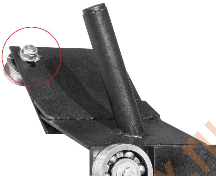
Рис 2. Регулировка зазора направляющей
