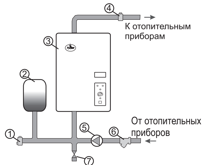
Рекомендуемая схема монтажа отопительной системы
