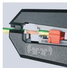
Прецизионное удаление изоляции 0,2 - 6,0 мм 2
