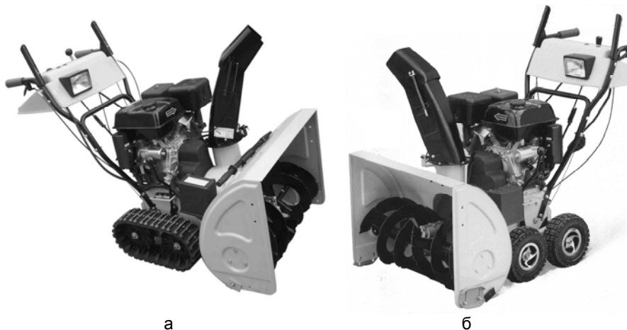
Рис. 1. Механизированные снегоуборщики с двигателем внутреннего сгорания а-MST901Q; б- MST1101Q.
