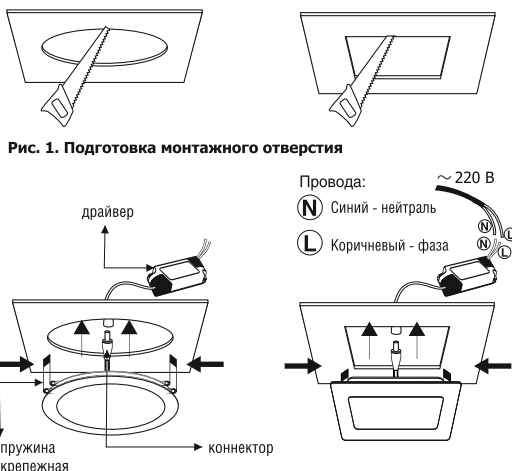
Рис. 2. Монтаж светильника
