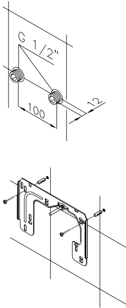
рис. 3 Установка прибора
