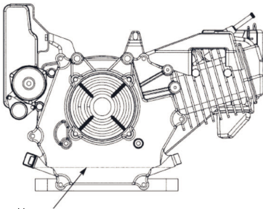
Уровень масла
