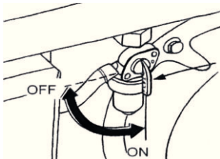
ТОПЛИВНЫЙ КРАН
