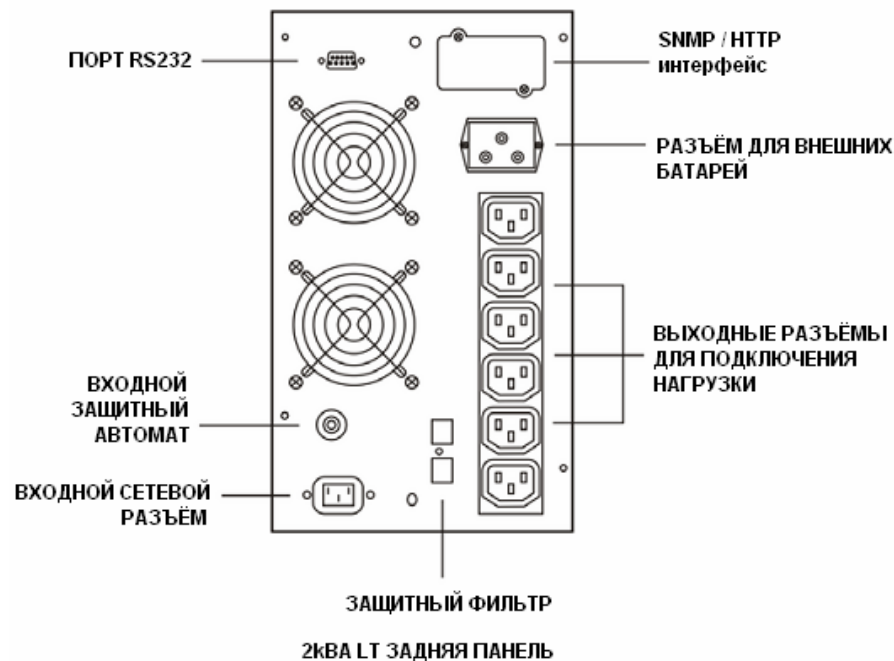
2кВА ЗАДНЯЯ ПАНЕЛЬ
