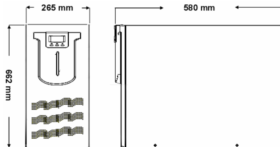
ПЕРЕДНЯЯ ПАНЕЛЬ
