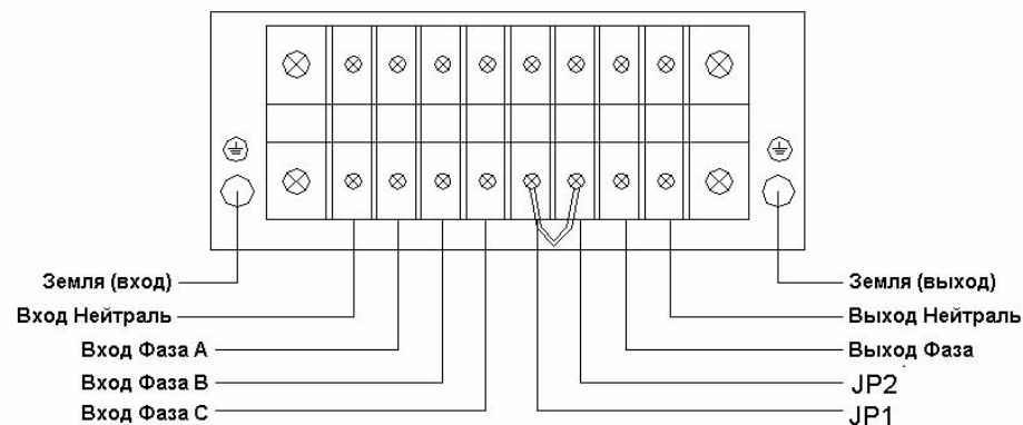
Клеммная панель Mega-Vision 10кВА(LT) 3ф/1ф.
