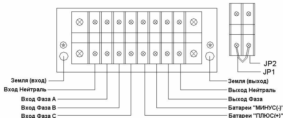
Клеммная панель Mega-Vision 15kVA LT / 20kVA LT 3ф/1ф.
