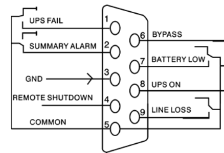
Рис. DB-9 Интерфейс AS400
