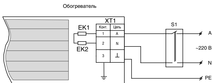
Рис. 2. Обогреватель ВИН-2.0
