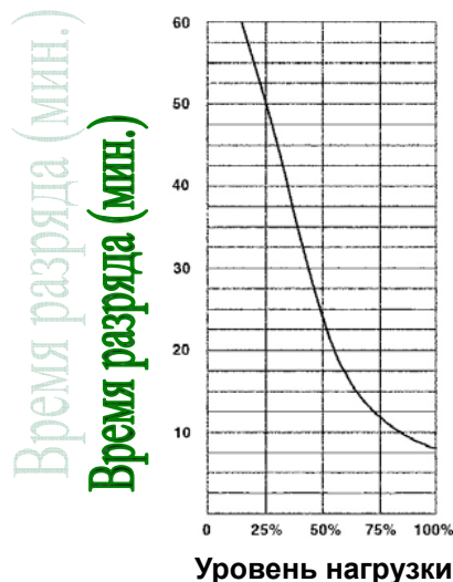
Зависимость времени резервирования от уровня нагрузки для MegaV6kVA
