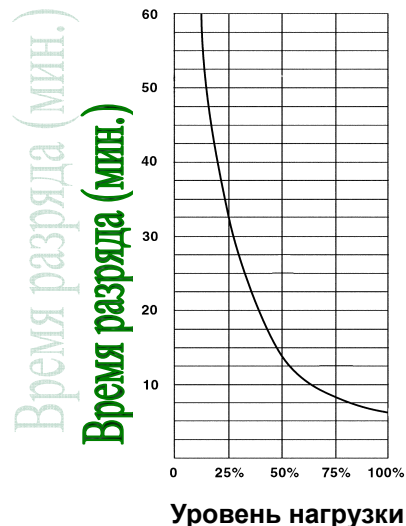
Зависимость времени резервирования от уровня нагрузки для MegaV10kVA
