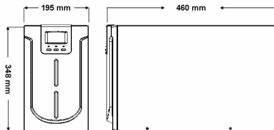
ПЕРЕДНЯЯ ПАНЕЛЬ
