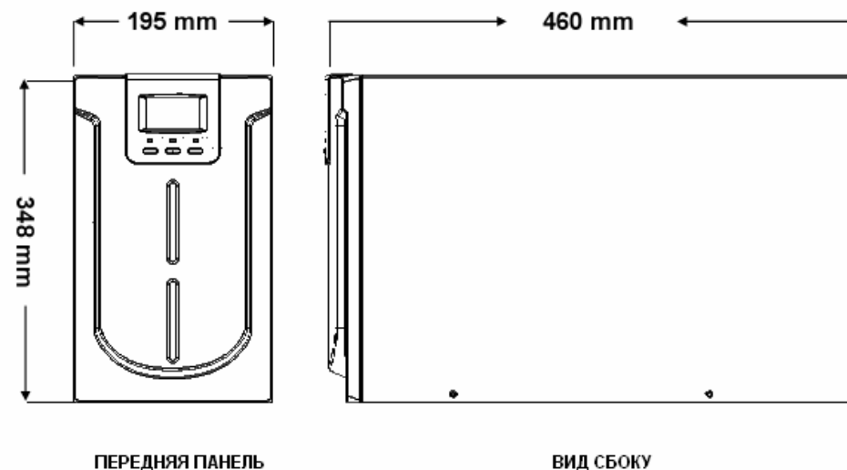
4-2-3 3кВА Стандартный корпус (Tower)
