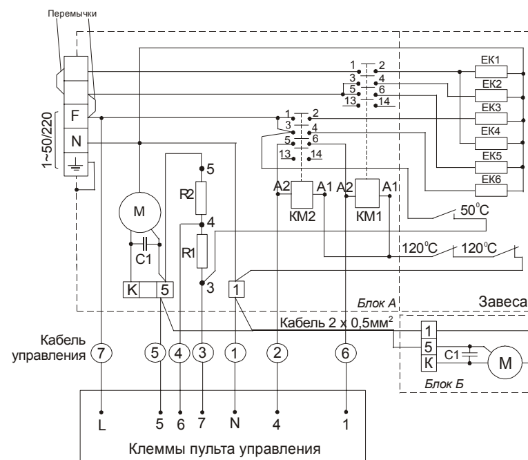
Рис. 5. Электрическая схема пульта управления
