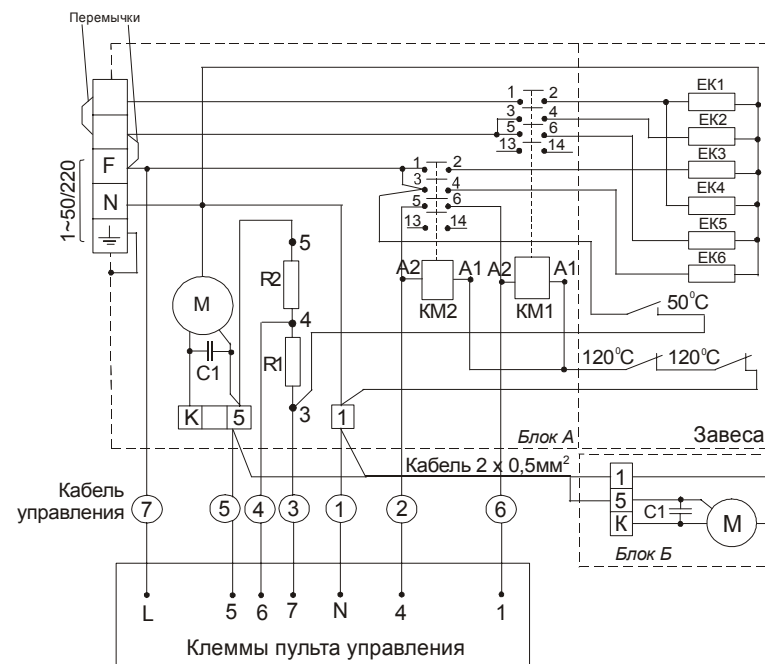
Рис. 5. Электрическая схема пульта управления
