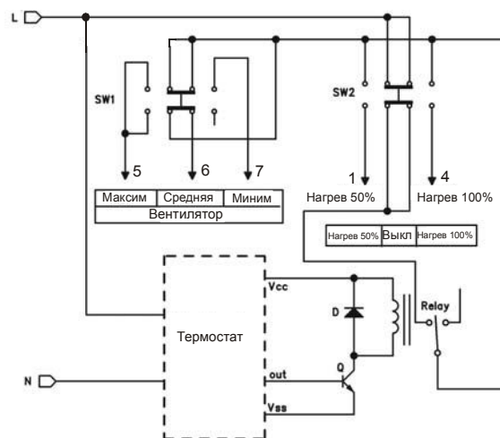
Рис. 5. Электрическая схема пульта управления
