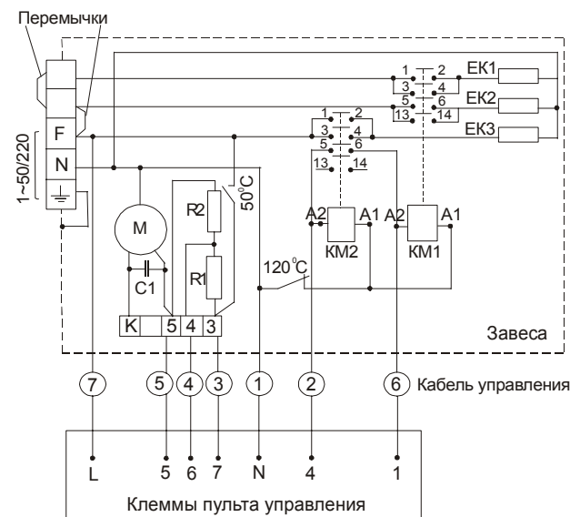
Рис. 1. Электрическая схема КЭВ-6П221Е
