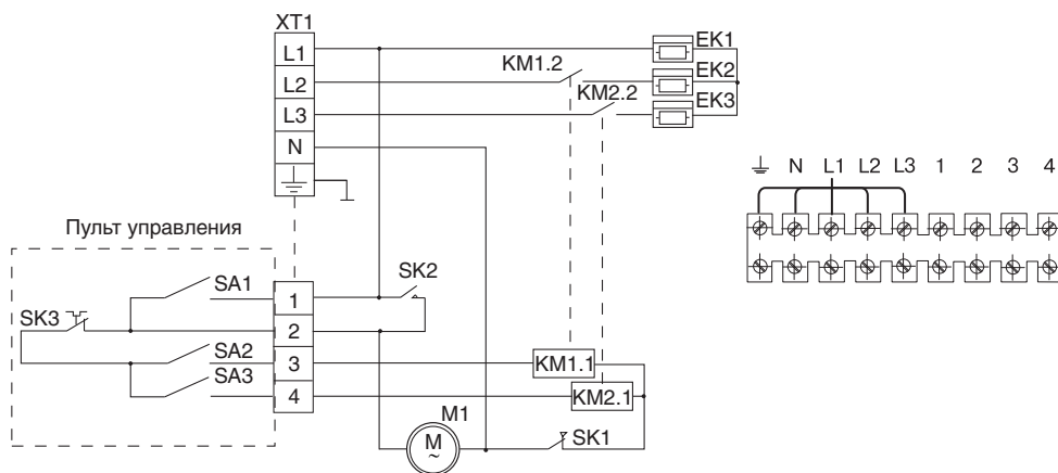
Рис. 3. Принципиальная схема BHC-3.000TR.
