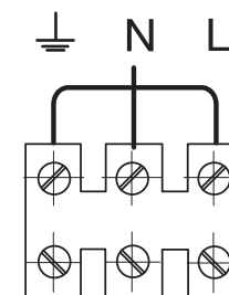
Рис. 3. Схема электрическая ВНЧ-5 SB(N)
