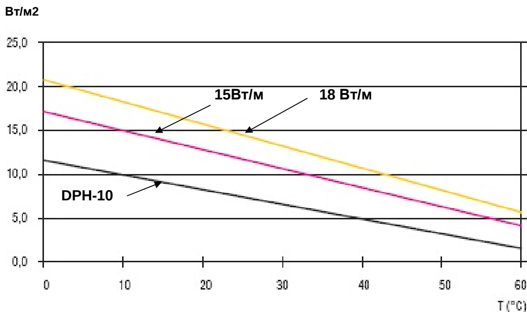
Рис. 1. Характеристика тепловыделения нагревательного кабеля Devi-Pipeheat™ DPH-10 (зависимость удельной мощности «сухого» кабеля от температуры окружающей среды)
