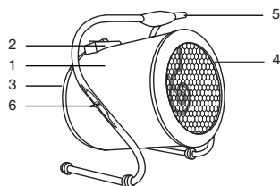
Рис. 1 Устройство прибора
