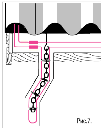
Цепь для фиксации кабеля в вертикальной водосточной трубе
