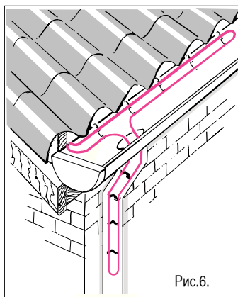
Крепление пластиковое для фиксации кабеля на цепи в трубе
