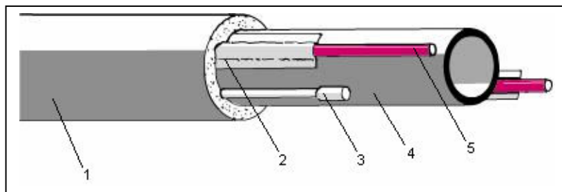
Рис. 5. Монтаж нагревательного кабеля Deviflex™ DTIP-10 на водопроводных трубах.
