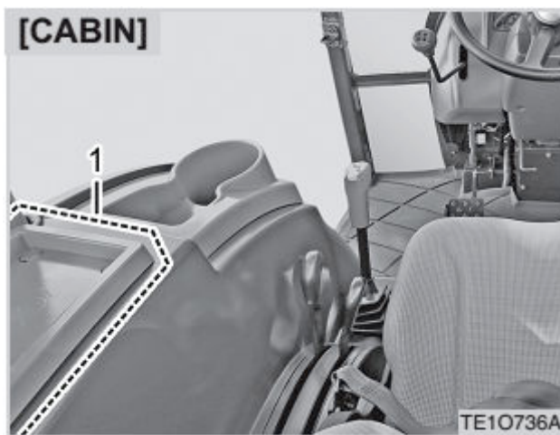
(1) Плавкие предохранители
