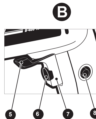
Рисунок В — элементы управления дрелью.
