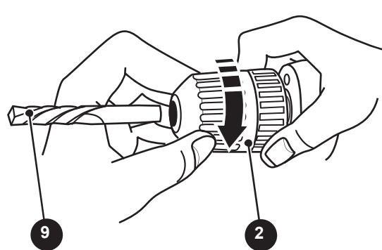
Рисунок С — установка сверла в быстрозажимной патрон.
