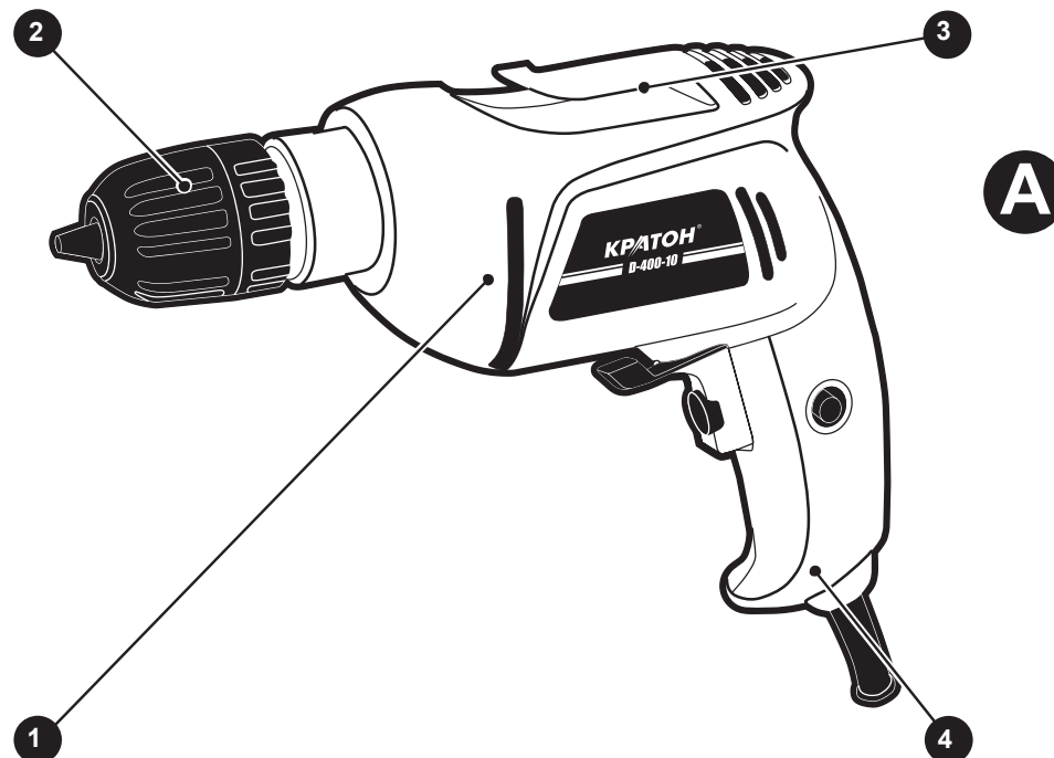
Рисунок А — общий вид дрели.
