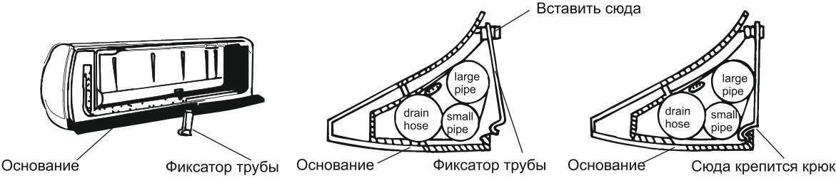
А. Вставьте фиксатор трубы в разъем.
