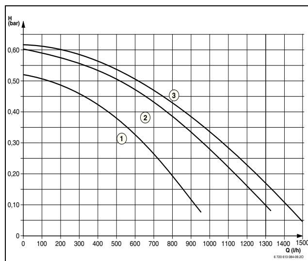
Рис 41 Характеристики насосов при ZSC/ZWC 35-3 (без монтажной соединительной панели)
