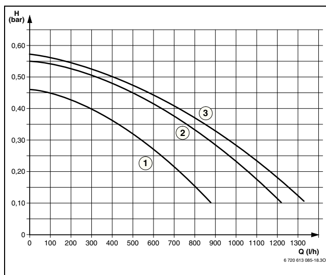
Рис 40 Характеристики насосов при ZWC 28-3 (без монтажной соединительной панели)
