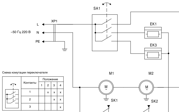
Рис. 4. Схема электрическая BHC-9.000SR
