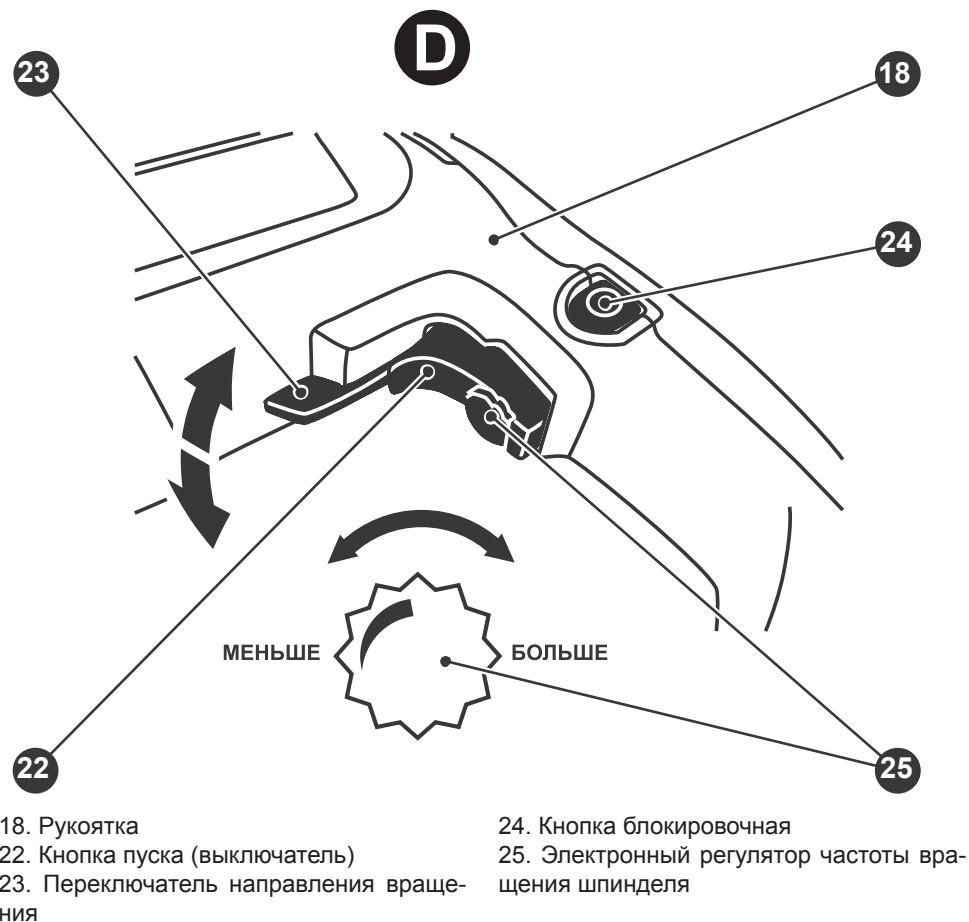
Рисунок D — элементы управления и регулирования перфоратора.
