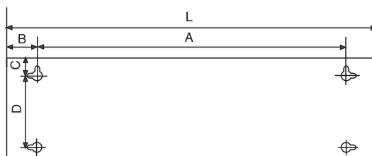
Рис. 5 Схема задней пластины завес
