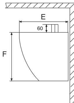
Рис. 6 Габаритные размеры завес
