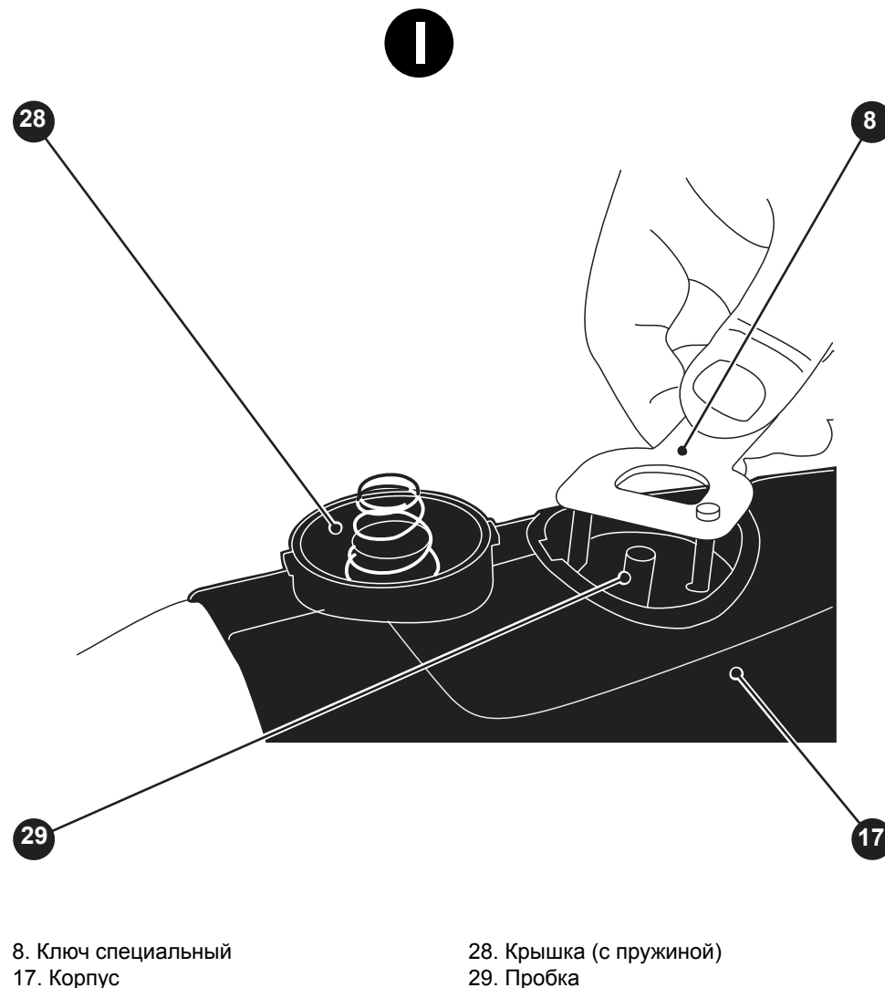
Рисунок I — подготовка перфоратора к заполнению смазкой редуктора.
