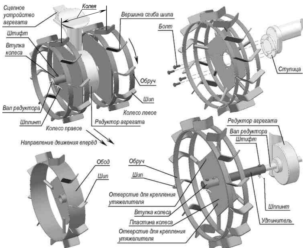
Рис. 1 Установка колёс на агрегат
