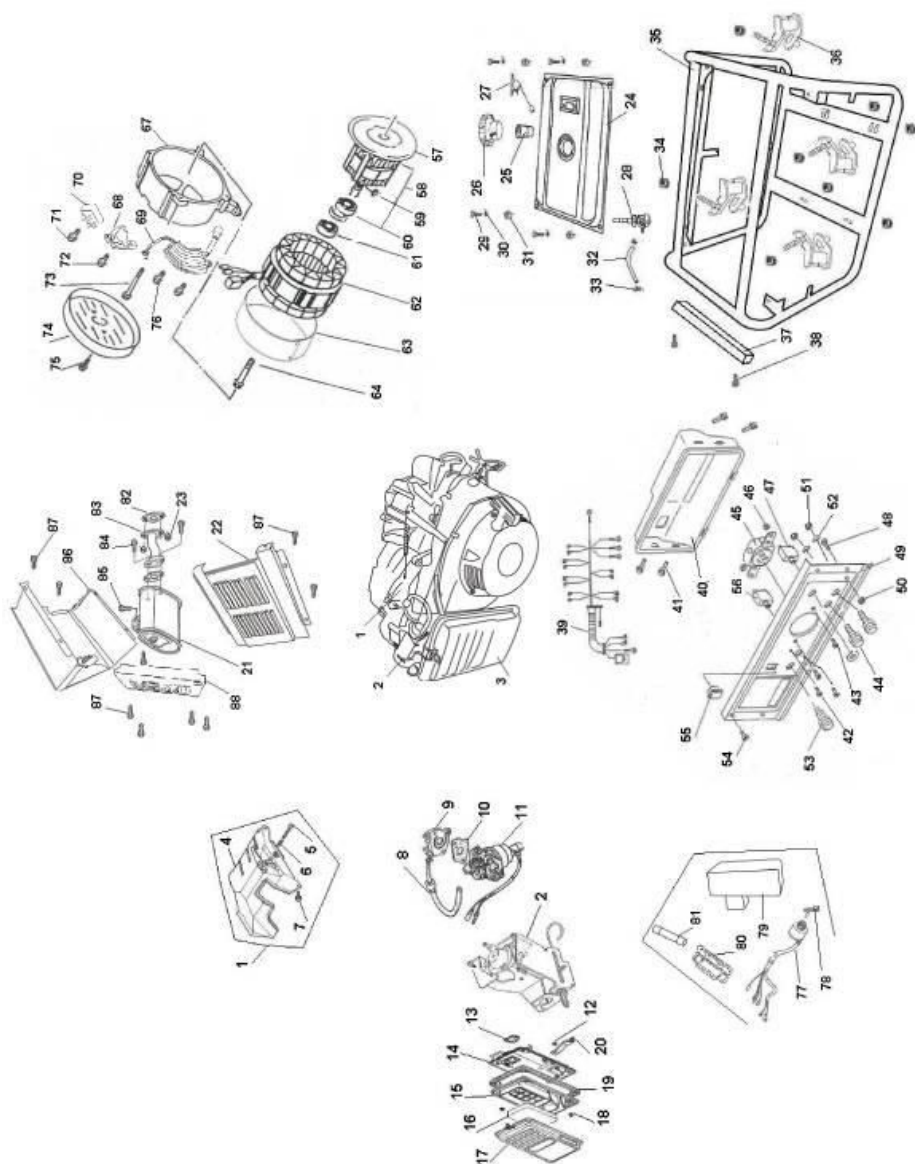
СХЕМА УСТРОЙСТВА И СБОРКИ ГЕНЕРАТОРОВ MG 4700, MG 6700E1
