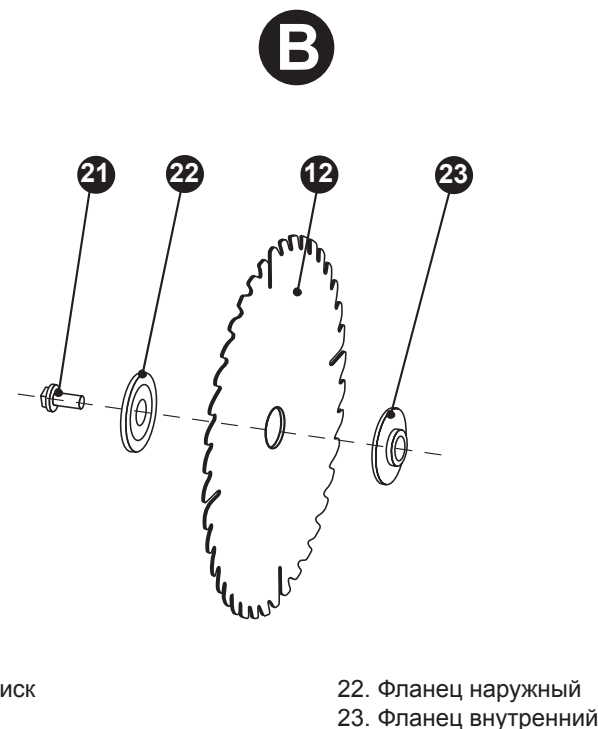
Рисунок В — элементы крепления пильного диска.
