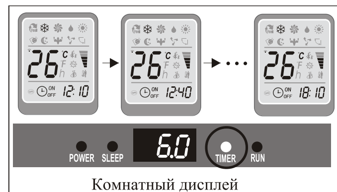
Комнатный дисплей
