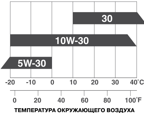
Температурный диапазон применяемости масел по классификации SAE
