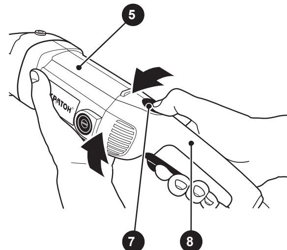
Рисунок Ф — установка необходимого положения поворотной рукоятки.
