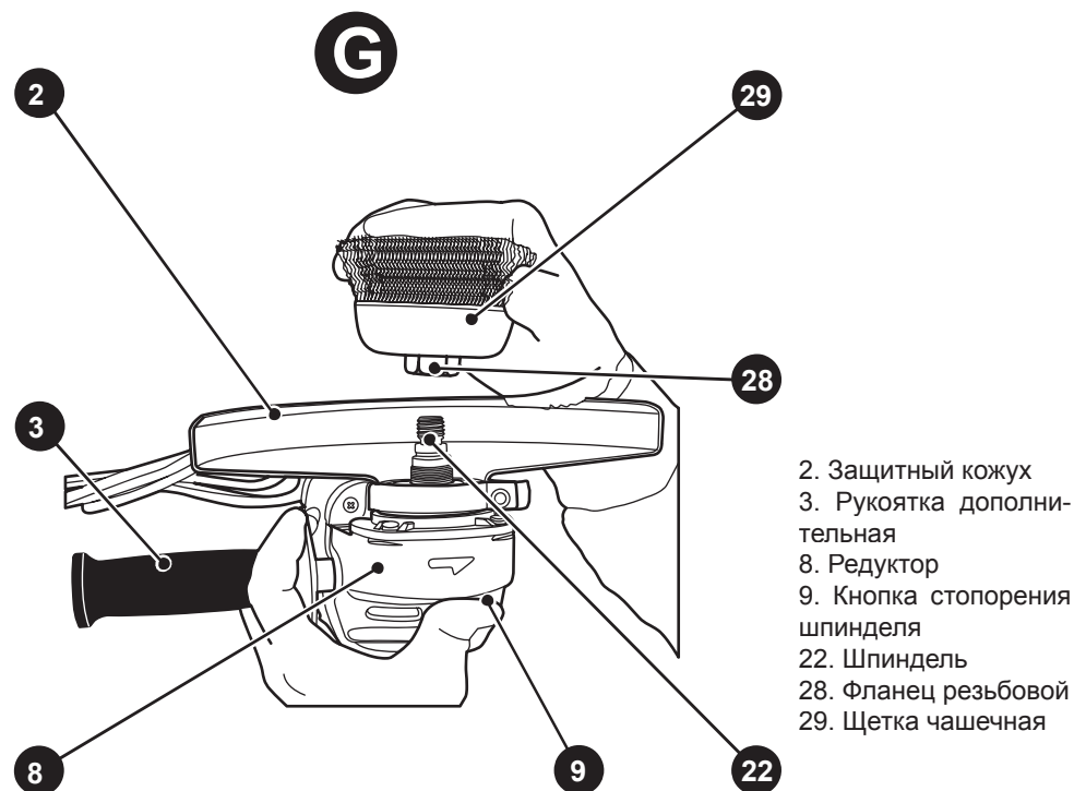
Рисунок G — установка и крепление чашечной щетки.
