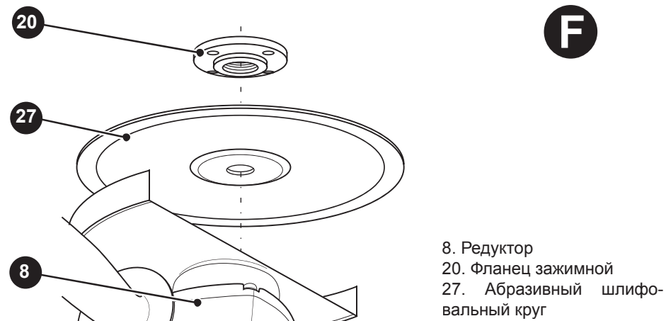
Рисунок F — установка и крепление абразивного шлифовального круга.
