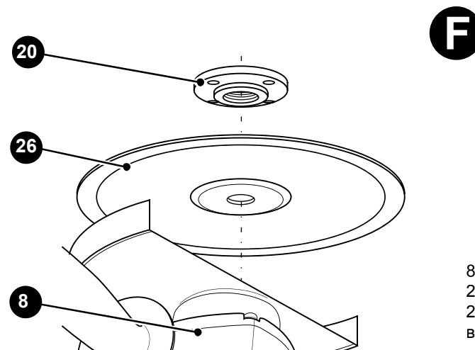
Рисунок F — установка и крепление абразивного шлифовального круга.
