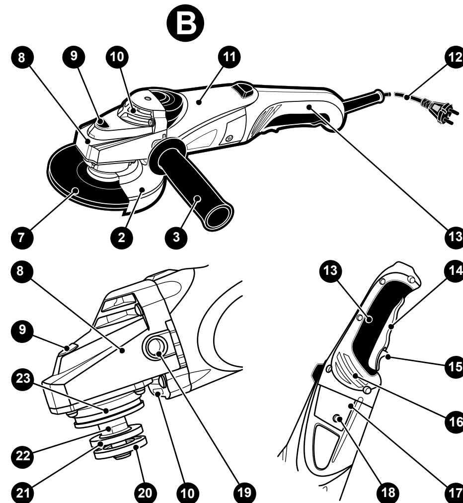
2. Защитный кожух 3. Рукоятка дополнительная 7. Абразивный отрезной круг 8. Редуктор 9. Кнопка стопорения шпинделя 10. Продувочные отверстия 11. Корпус 12. Кабель электропитания с вилкой 13. Рукоятка 14. Выключатель
