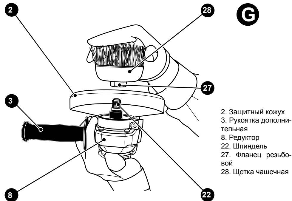
Рисунок G — установка и крепление чашечной щетки.
