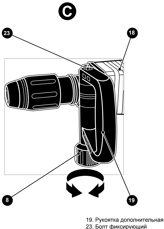
Рисунок С — регулирование положения дополнительной рукоятки молотка.
