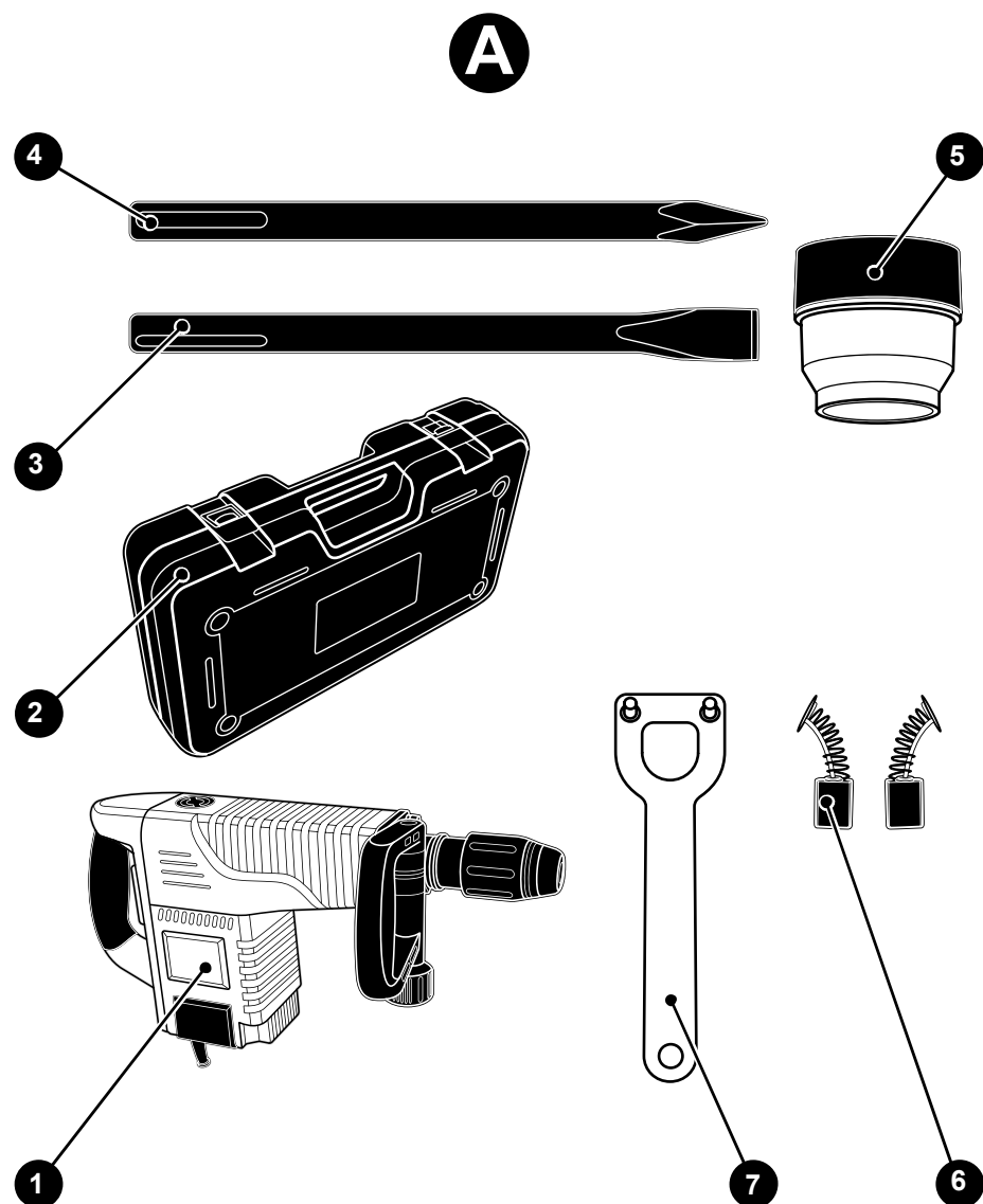
Рисунок А — комплектность молотка. Дополнительно смотри таблицу 2.
