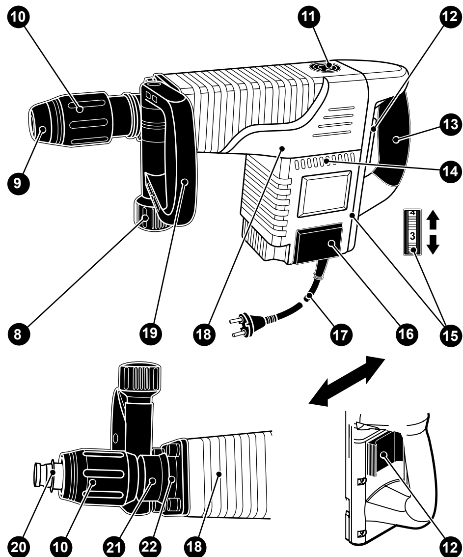
Рисунок В — общий вид молотка.
